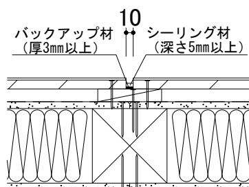
＜バックアップ材を用いた伸縮目地の納まり例＞
